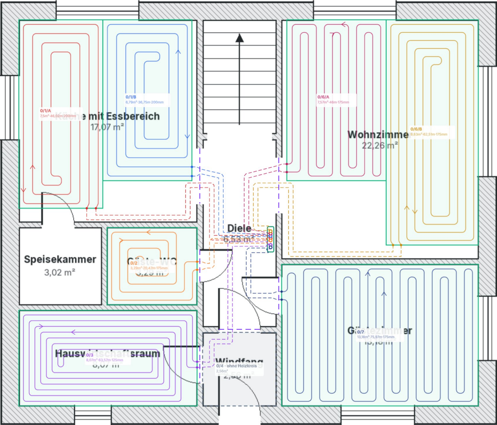
ERDGESCHOSS
